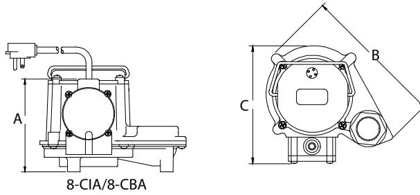
8-CIA/8-CBA
