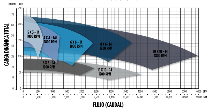
Curva de Familia Serie HC 14"
