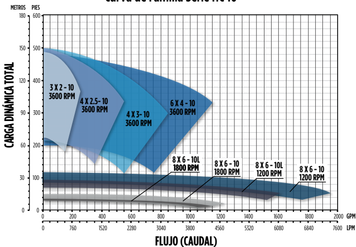
Curva de Familia Serie HC 10"
