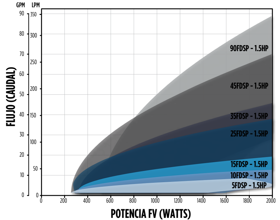
Curva de Rendimiento Serie FHOTON™ SolarPAK 1.5 HP
