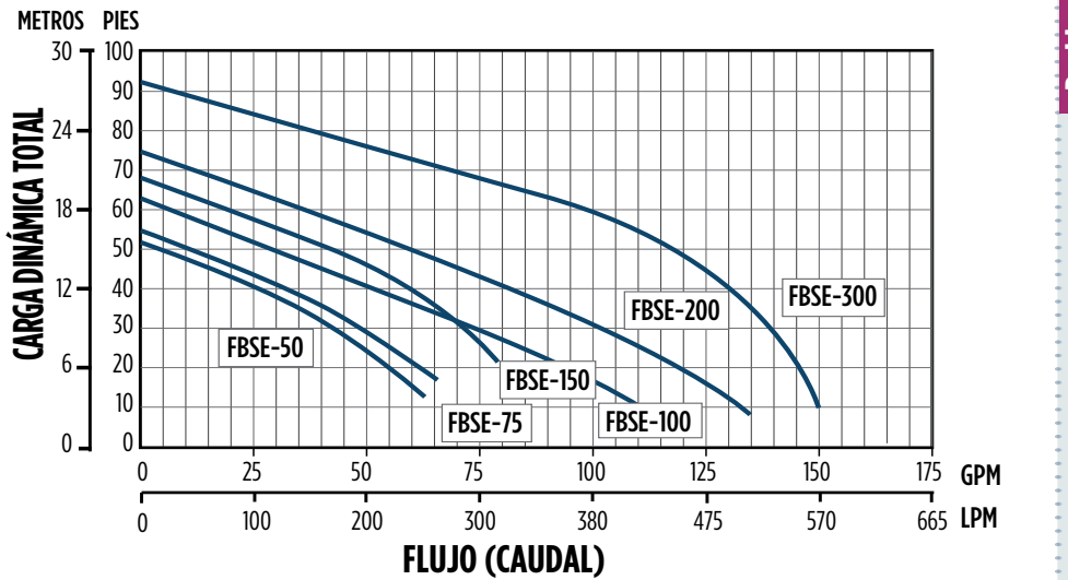
Curva de Rendimiento de la Serie FBSE
