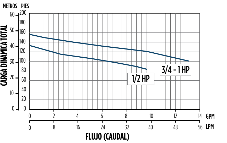
Curva de Rendimiento de la Serie SWJ
