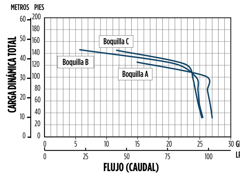
Curva de Rendimiento de la Serie Versajet 1.5 HP
