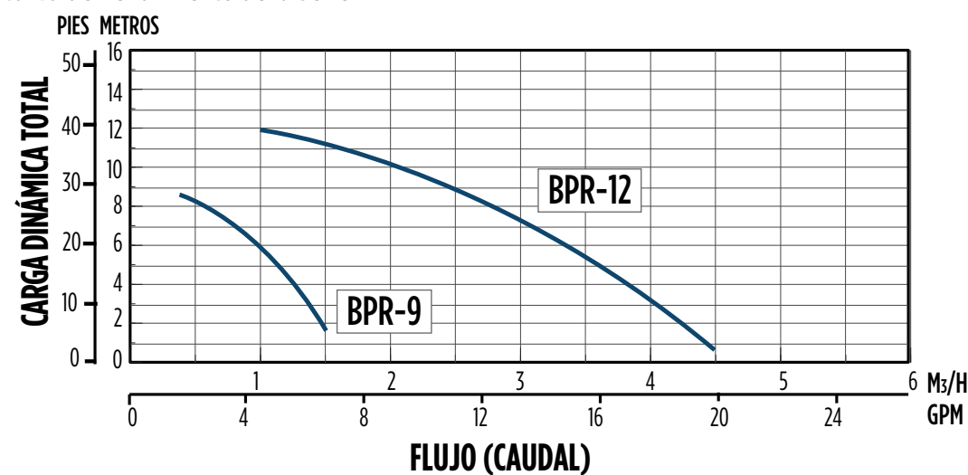
Curva de Rendimiento de la Serie BPR
