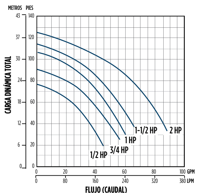
Curva de Rendimiento de la Serie FCE
