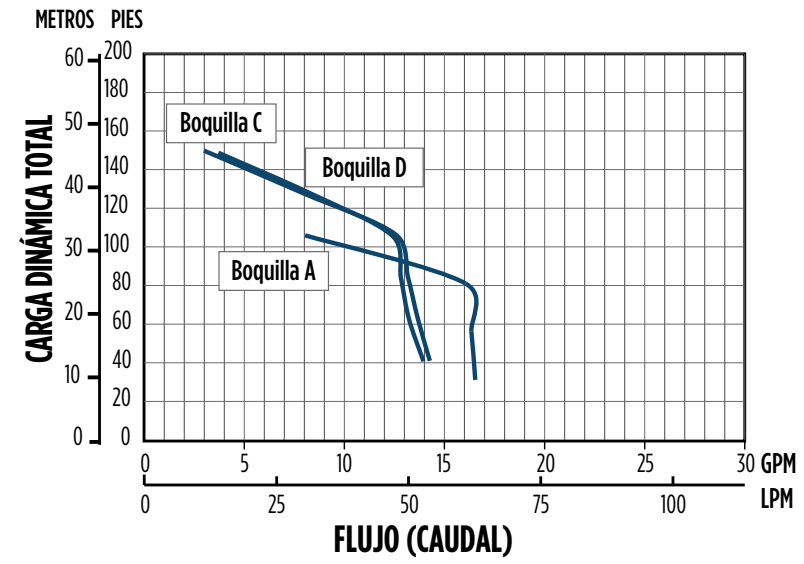
Curva de Rendimiento de la Serie Versajet 1 HP
